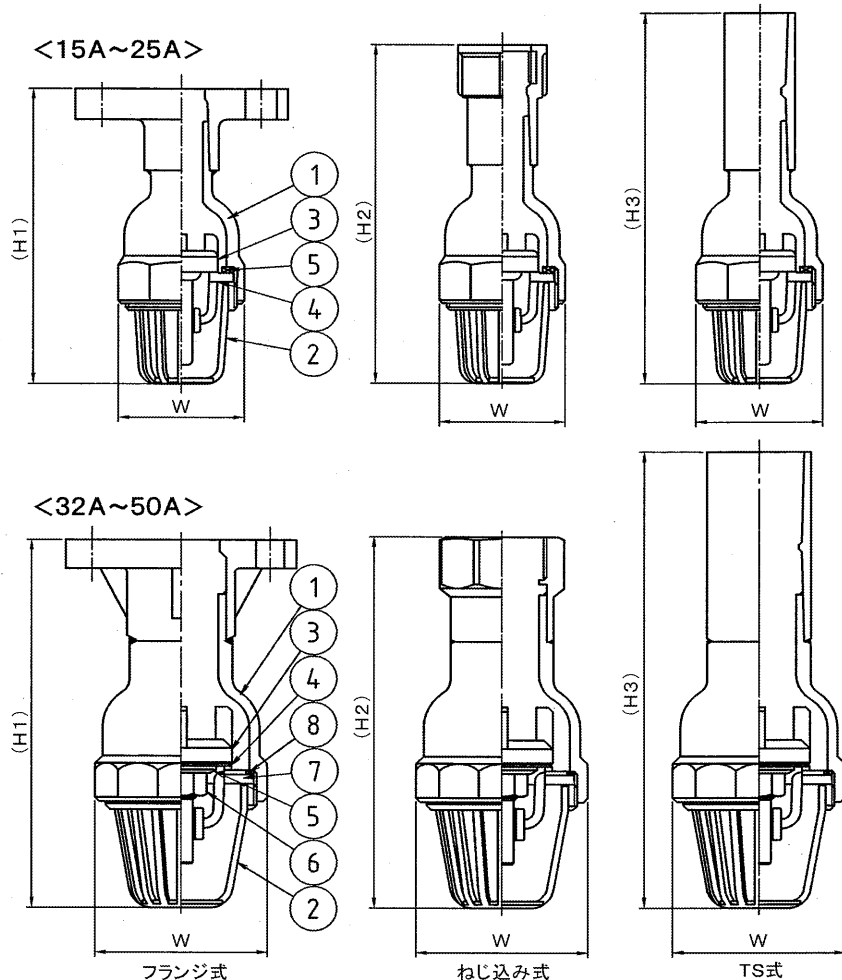
<M401型寸法表>
