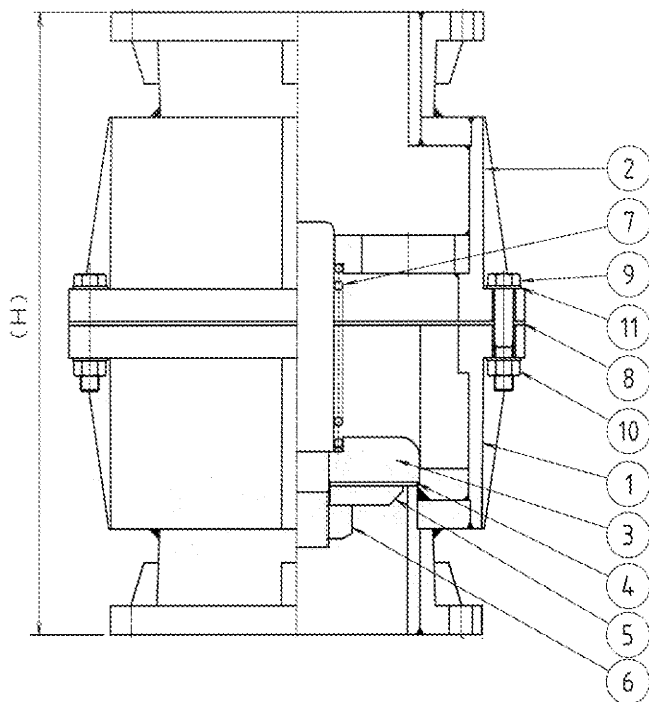
<DS404型 寸法表>
