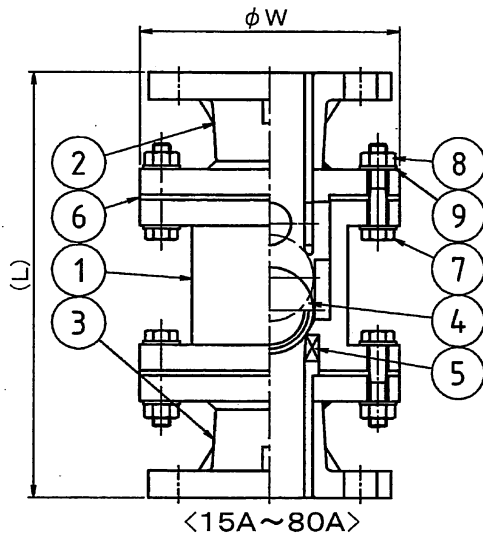
<S4002型 寸法表>
